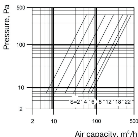
136-05 & 136-25 (125mm)
